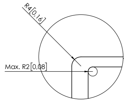
DETALLE F ESCALA 1 : 1
